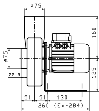
Ständerausführung ML
