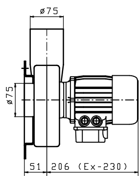
Flanschausführung MLF
