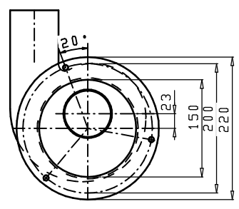
Flanschausführung MLF
